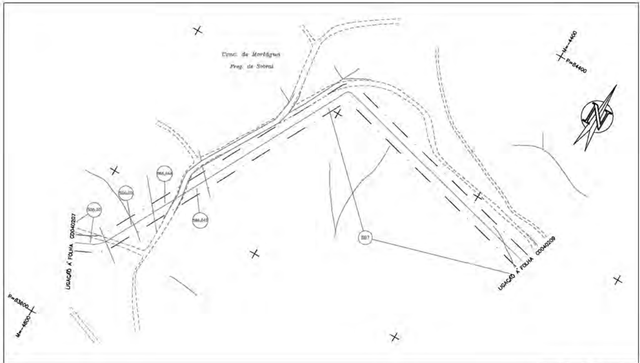
P-11000-DWG-CD-040208-REV.2
