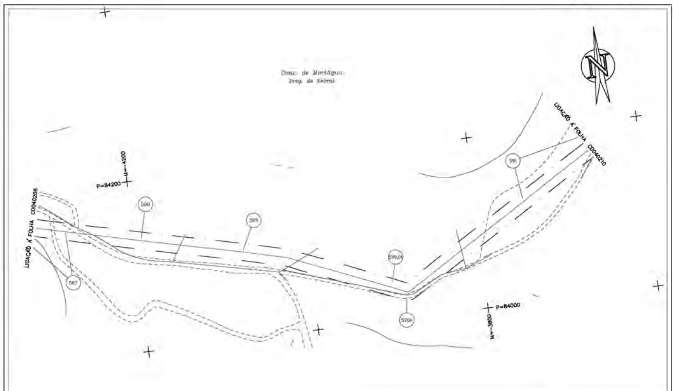
P-11000-DWG-CD-040208-REV.2
