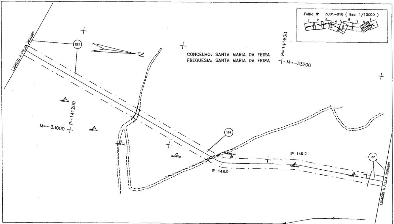
P-3001-DWG-CD-16.08-REV.2
