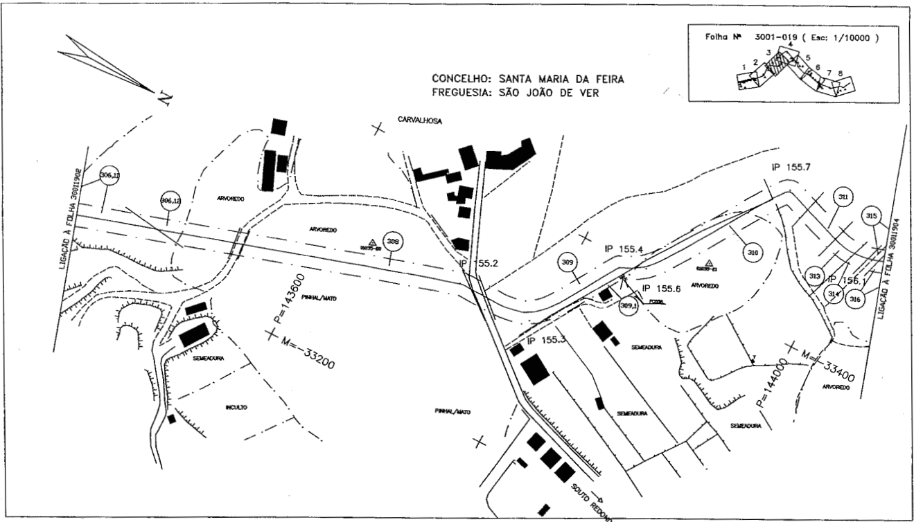
P-3001-DWG-CD-19.03-REV.2
