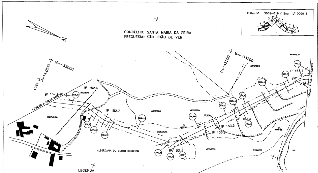
P-3001-DWG-CD-19.01-REV.2
