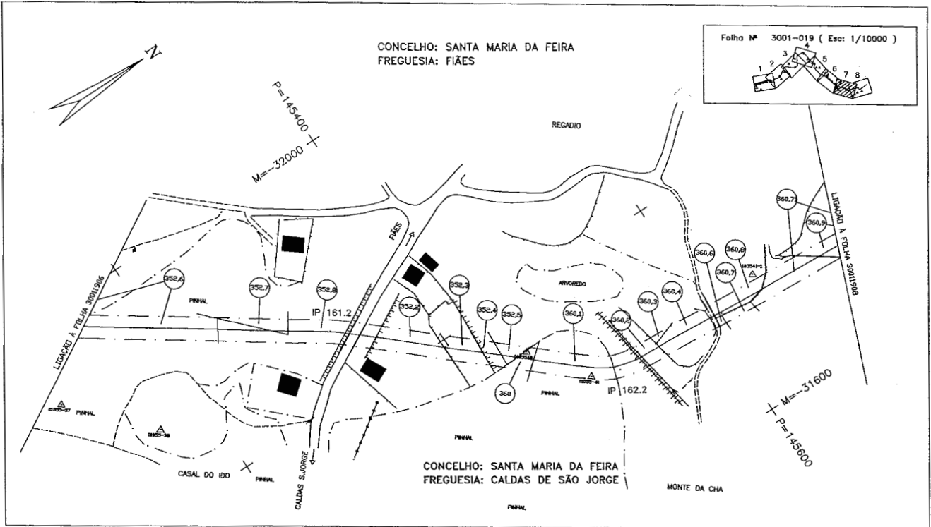
P-3001-DWG-CD-19.07-REV.2
