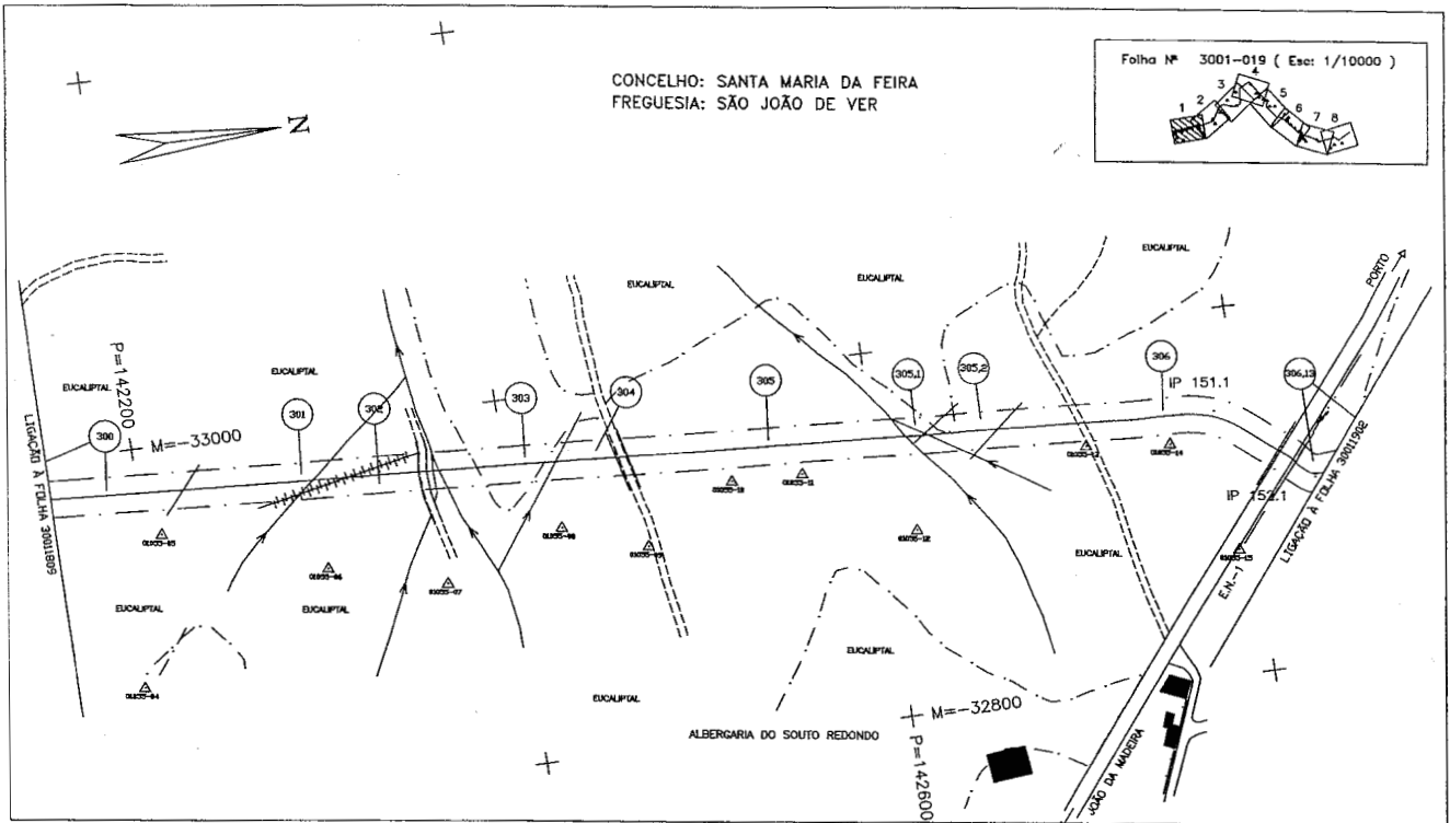
P-3001-DWG-CD-19.01-REV.2
