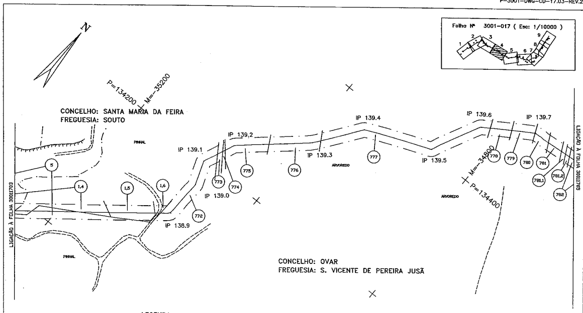
P-3001-DWG-CD-17.03-REV.2
